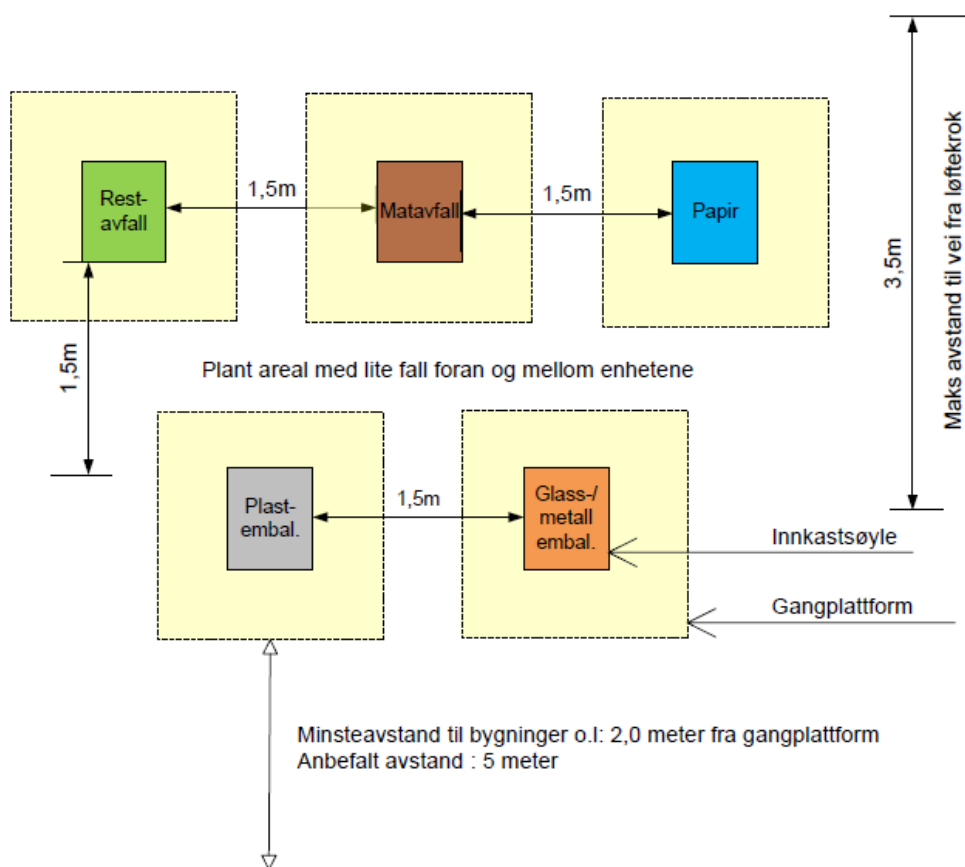
Figur 5-9: Eksempel på arrangement og plassbehov for helt nedgravd løsning for 20 boenheter.
